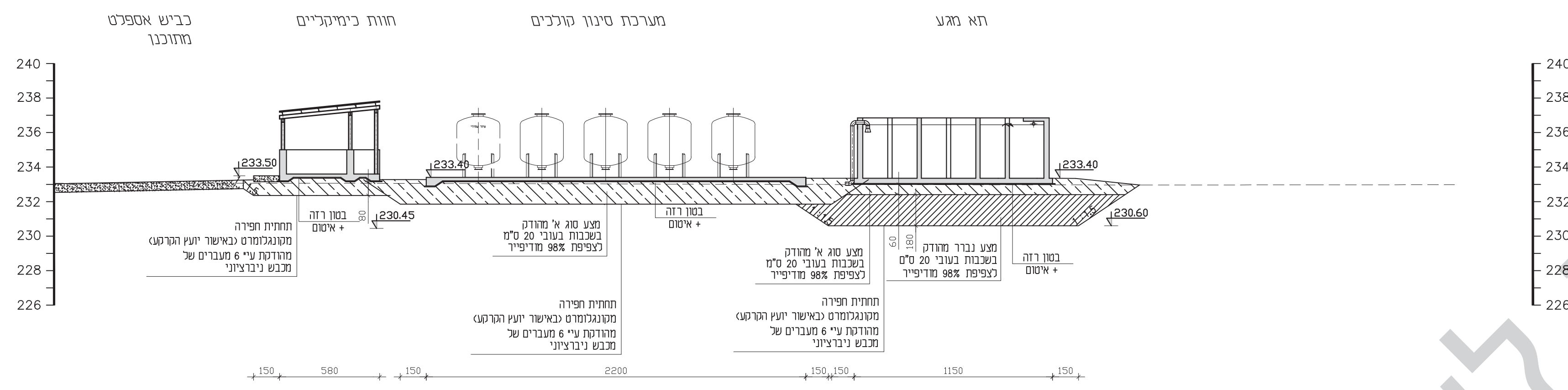
צתת D-D קב"צ 1:200
