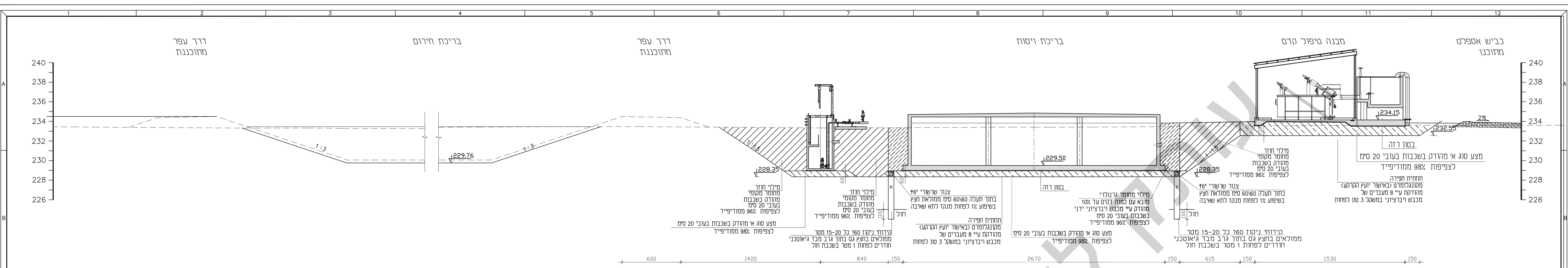
חתך A-A קב"ח 1:200
